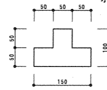
B 詳細図 S=1:5
