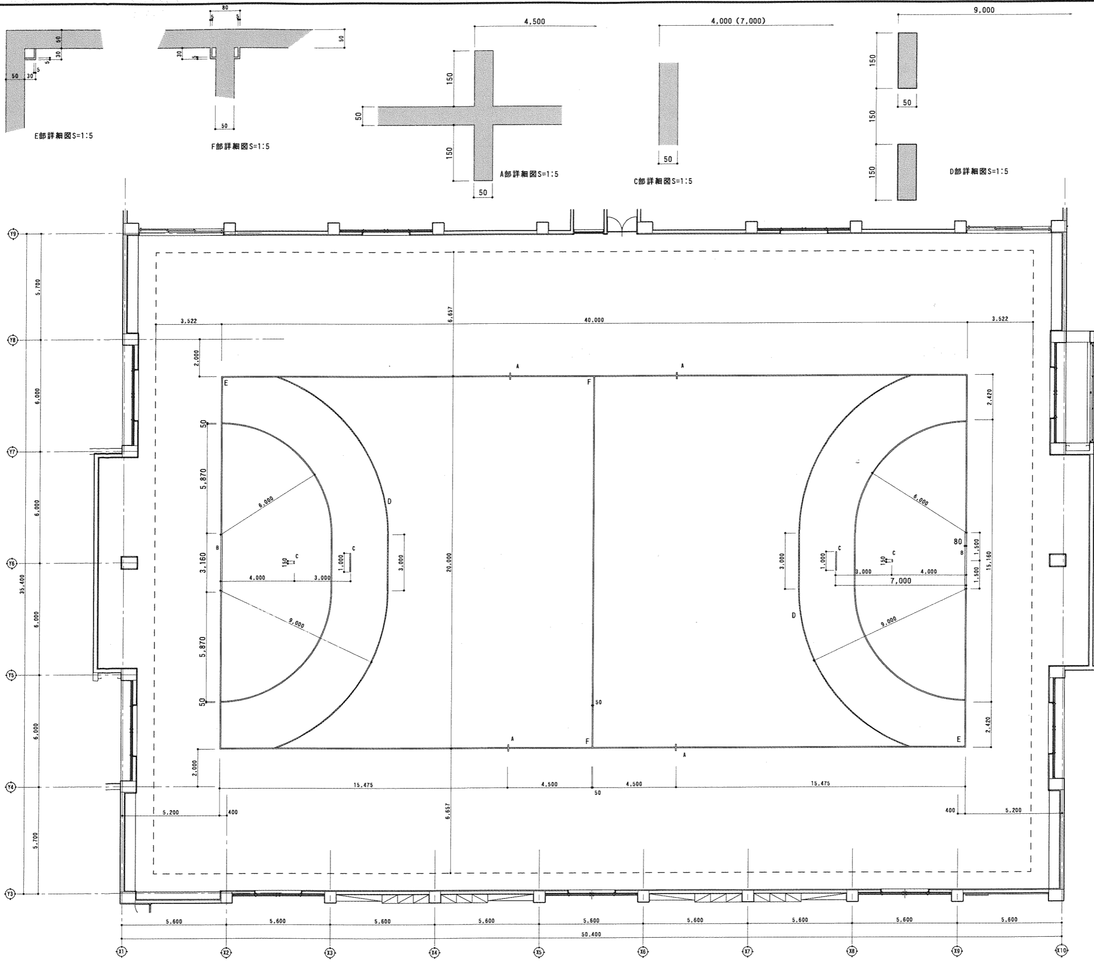
ハンドボールコートライン (全線) 1:100
